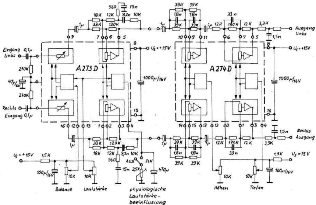
Schaltbild Lautstärke-, Balance-, Höhen- und Tiefenregler
